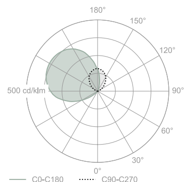
Krzywa światłości
