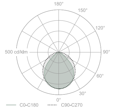
Krzywa światłości
